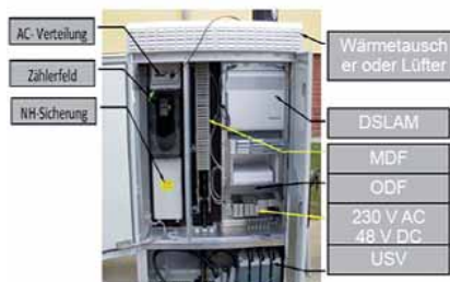
Technischer Aufbau eines sog. DSLAM
