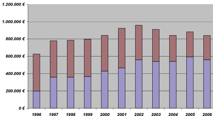
Die Defizitentwicklung für den DINGO (blau dargestellt) und das Parkdeck am Auenweg (rot dargestellt) über die Jahre 1996 – 2006
