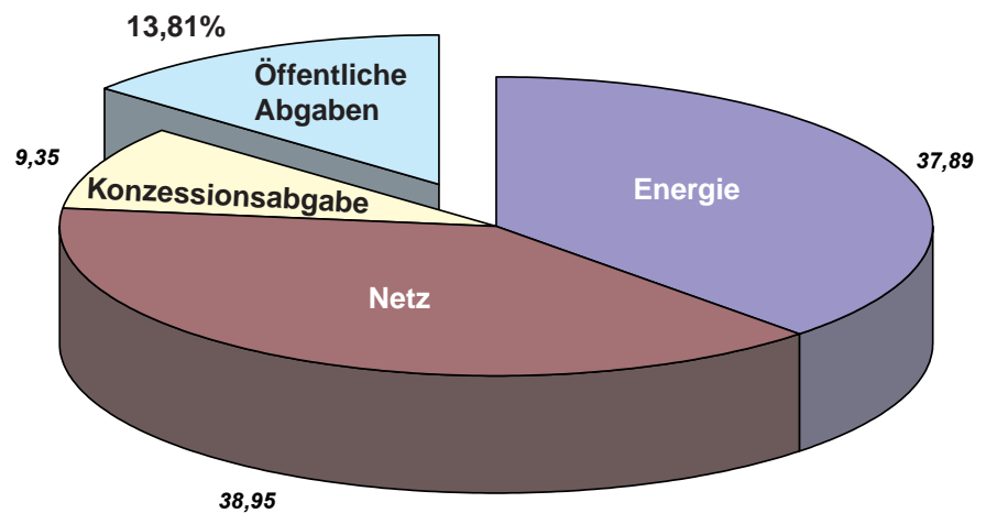
Zusammensetzung des Strompreises im Jahr 1998
